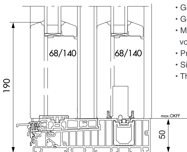
Profil im Querschnitt
